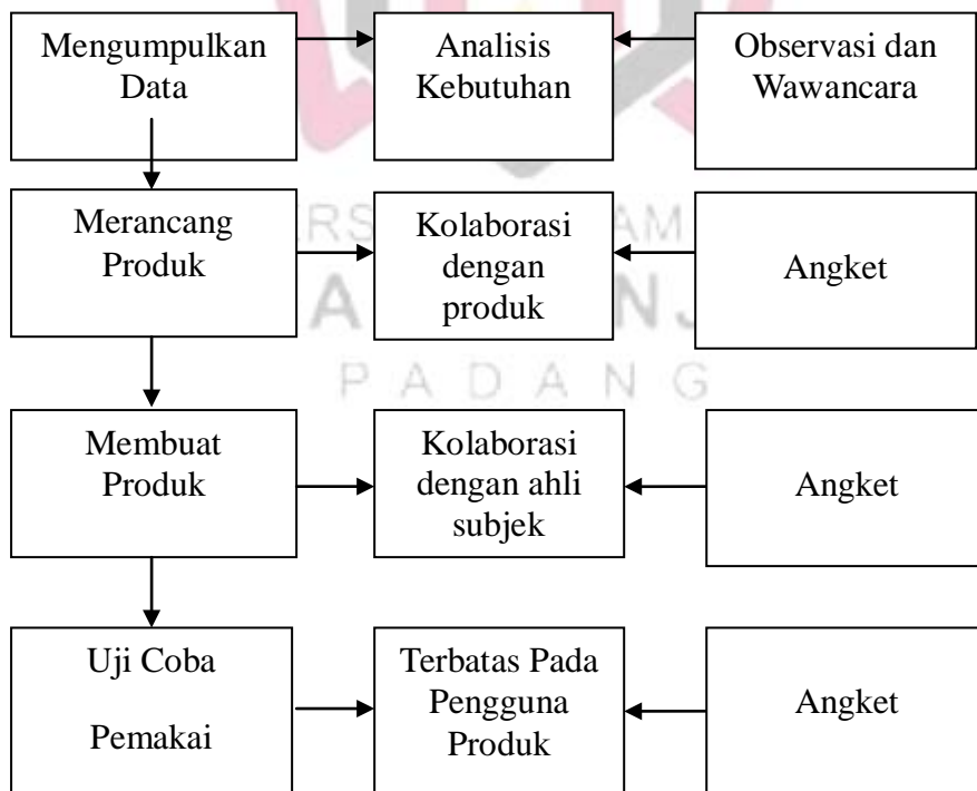
Gambar 1. Prosedur Pengembangan
